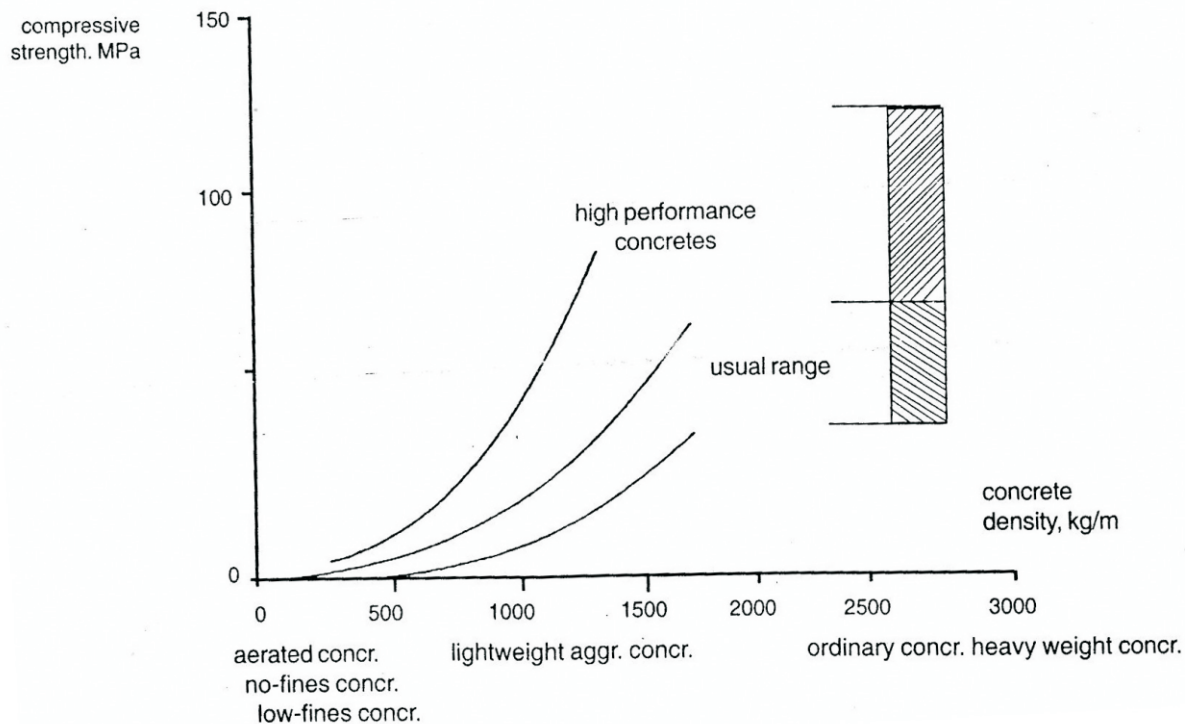
Gambar 2. Spektrum Berat dan Kekuatan Material Beton [3]
