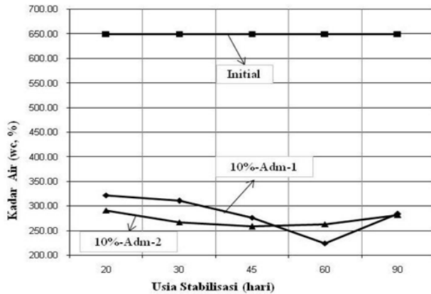
Gambar 5. Pengaruh usia stabilisasi terhadap nilai kadar air gambut yang distabilisasi
