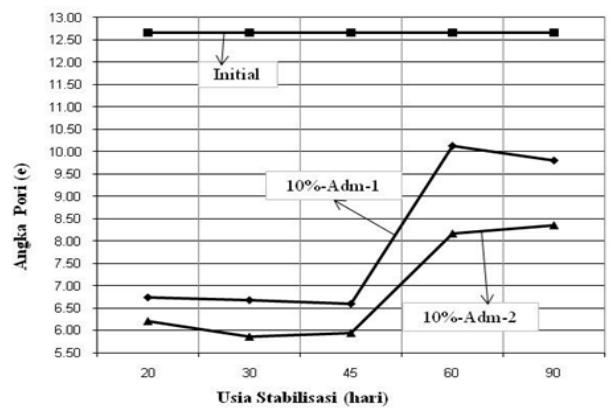
Gambar 7. Pengaruh usia stabilisasi terhadap nilai angka pori gambut yang distabilisasi
