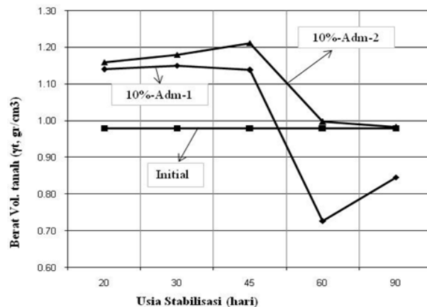
Gambar 4. Pengaruh usia stabilisasi terhadap nilai berat volume tanah gambut yang distabilisasi
