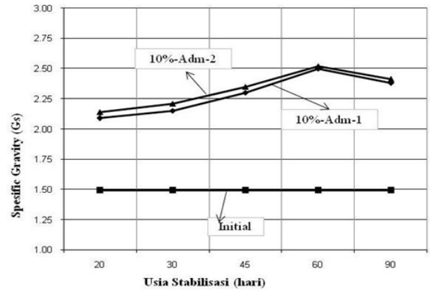
Gambar 6. Pengaruh usia stabilisasi terhadap nilai berat jenis (Gs) gambut berserat yang distabilisasi
