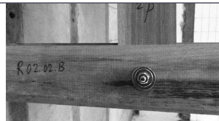
Gambar 12. Benda uji sambungan kayu Rengas
