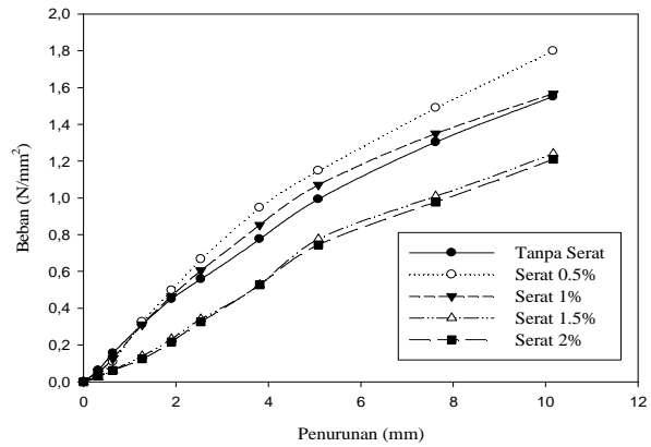
Gambar 11. Grafik hubungan antara Beban dengan penurunan (panjang serat=15mm)
