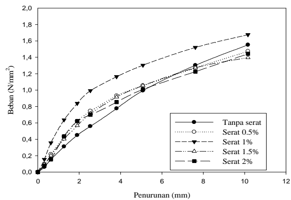
Gambar 12. Grafik hubungan antara Beban dengan penurunan (panjang serat=20mm)
