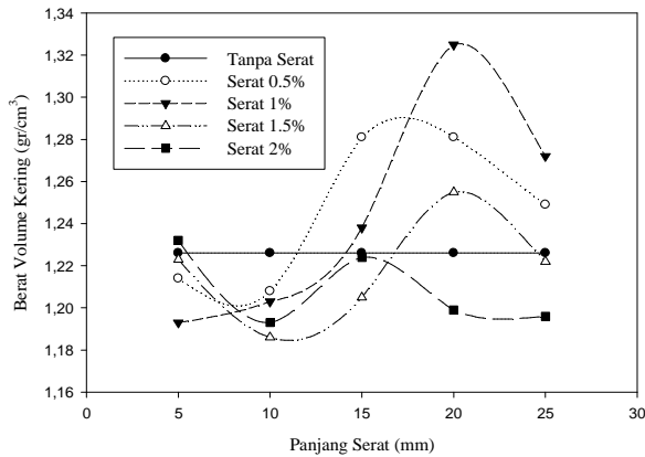
Gambar 8. Hasil uji pematidatan standard proctor lempung, trass, asetilen, variasi serat
